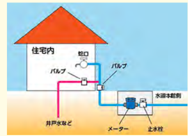
【クロスコネクション概要図】
